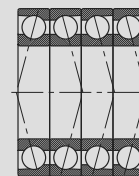
QBT Combinação da disposição em O e em Tandem
