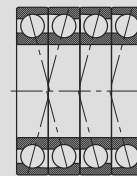
QFT Combinação da disposição em X e em Tandem
