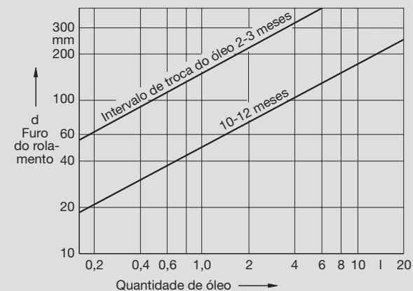
▼ Quantidade de óleo e intervalos para a troca, dependendo do furo do rolamento
