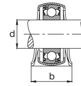
SB2 combinado com 762..2RSR
