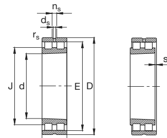
NN30ASK (conicidade 1:12)
