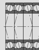
QBC Disposição em O
