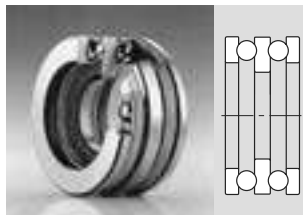
Rolamento axial de esferas de escora dupla
