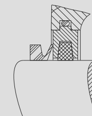
Vedação de feltro + anel V
