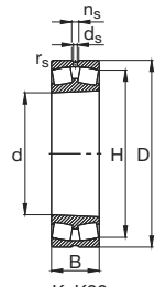
K, K30 Furo cônico (cone 1:12 ou 1:30)
