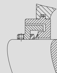
Vedação de labirinto + vedação de contato (Taconite)
