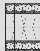
QFC Disposição em X
