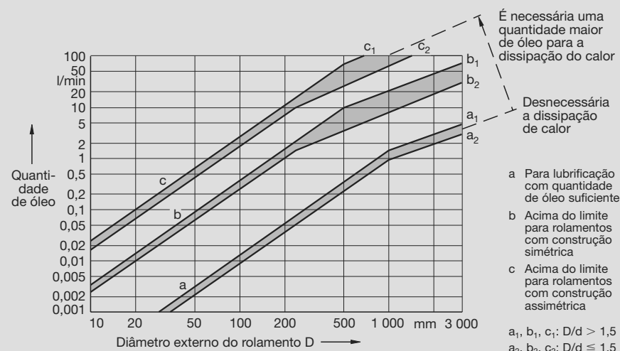
▼ Quantidades de óleo na lubrificação por recirculação
